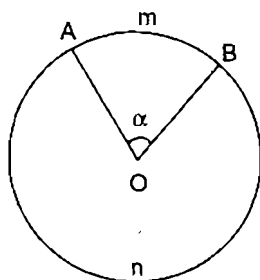
a) 0^\circ < \alpha < 180^\circ
