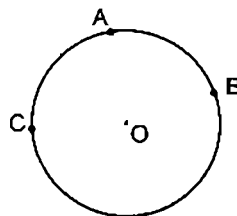
Hình 4. Điểm C nằm trên cung lớn AB
