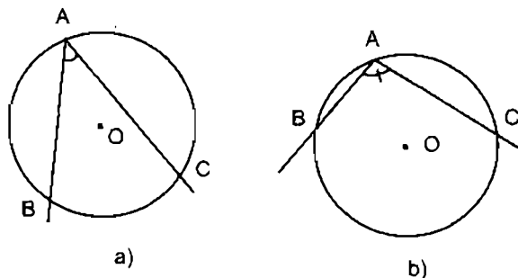
Hình 13. \widehat{BAC} là góc nội tiếp.
